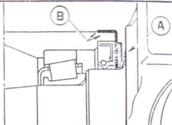
MONTAGGIO NUOVO ANELLO 110150 110150 NEW RING ASSEMBLY
